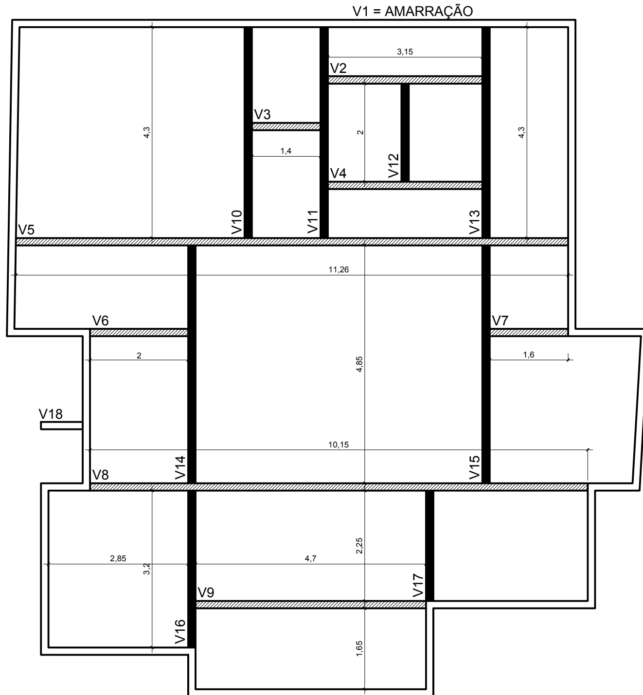
PLANTA BAIXA VIGA BALDRAME
