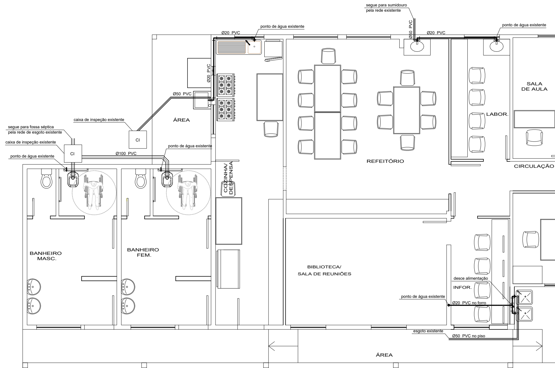
PROJETO HIDROSSANITÁRIO Escala 1/75
