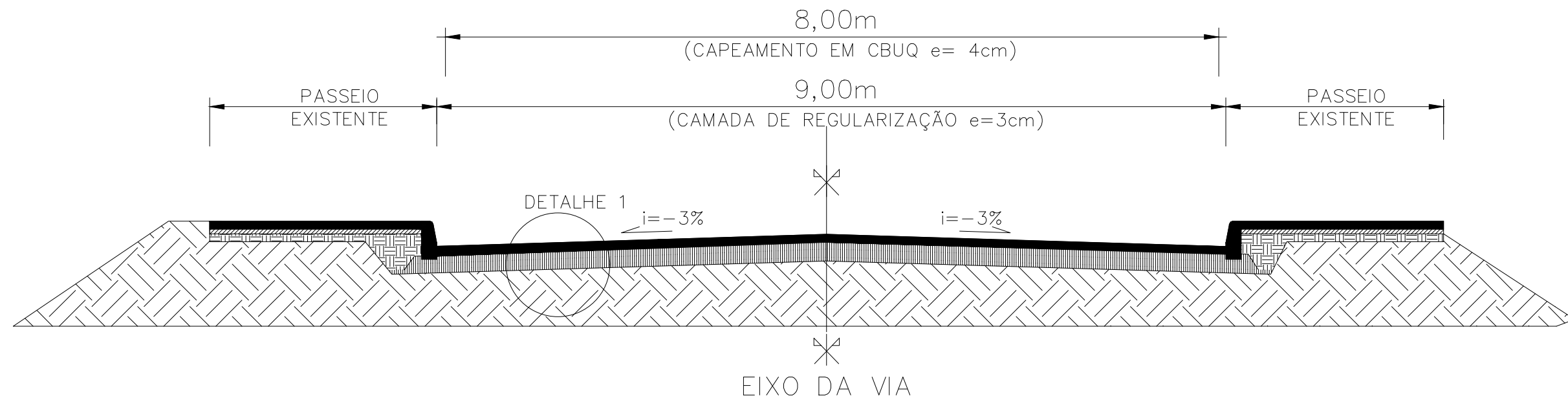
SEÇÃO TIPO DE CAPEAMENTO SEM ESCALA
