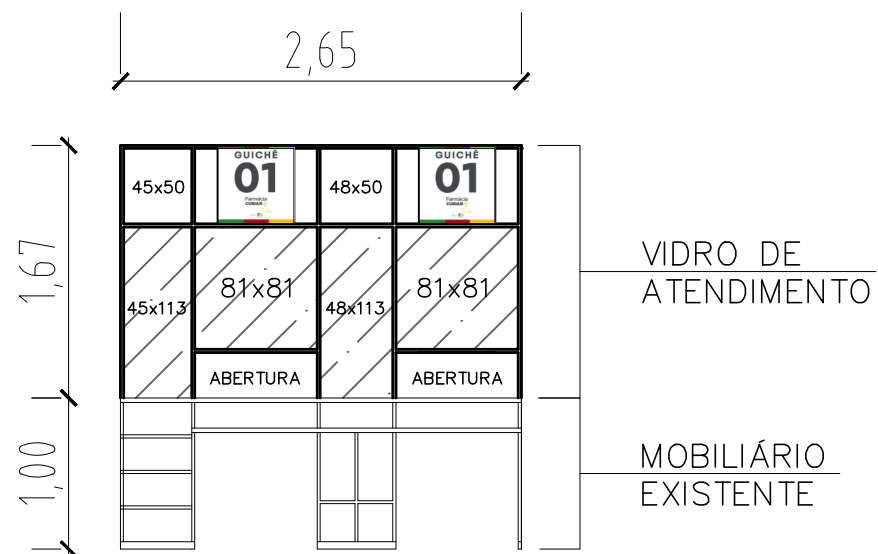
DET. 03 - GUICHÊS ESC: 1/50
