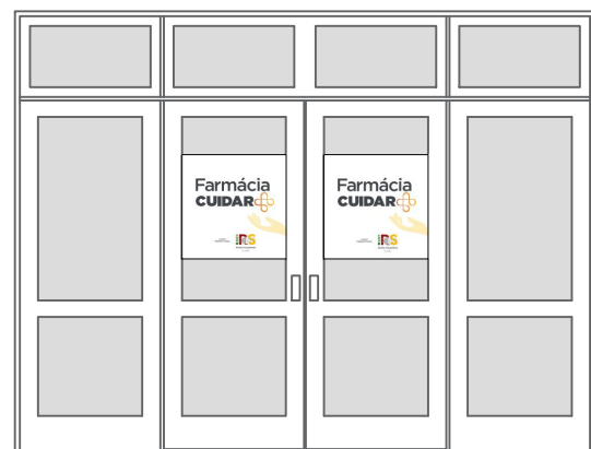
DET. 02 - PORTA ACESSO ESC: 1/50
