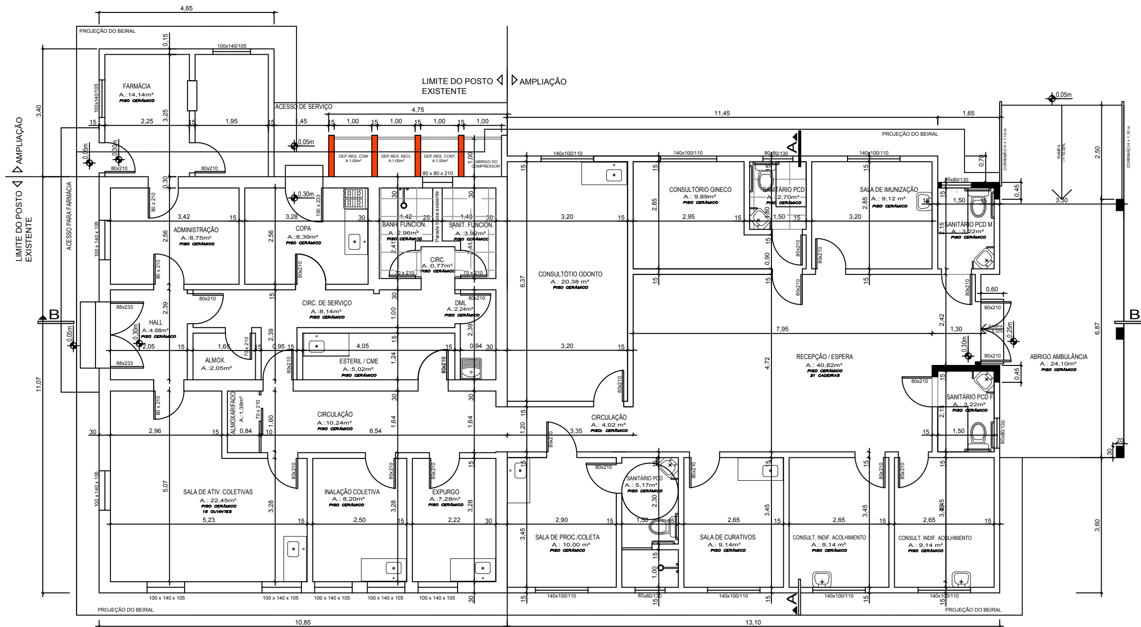
UNIDADE DE SAÚDE QUITÉRIA PLANTA BAIXA EXISTENTE COTADA ÁREA : 120,10 m 2
