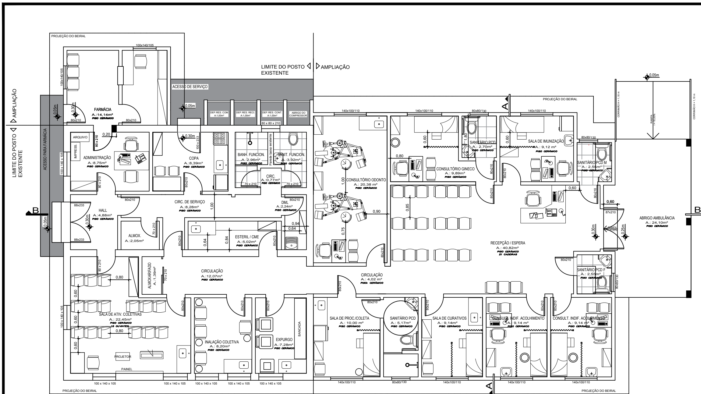
PLANTA BAIXA EXISTENTE MOBILIADA ÁREA : 120,10 m 2
