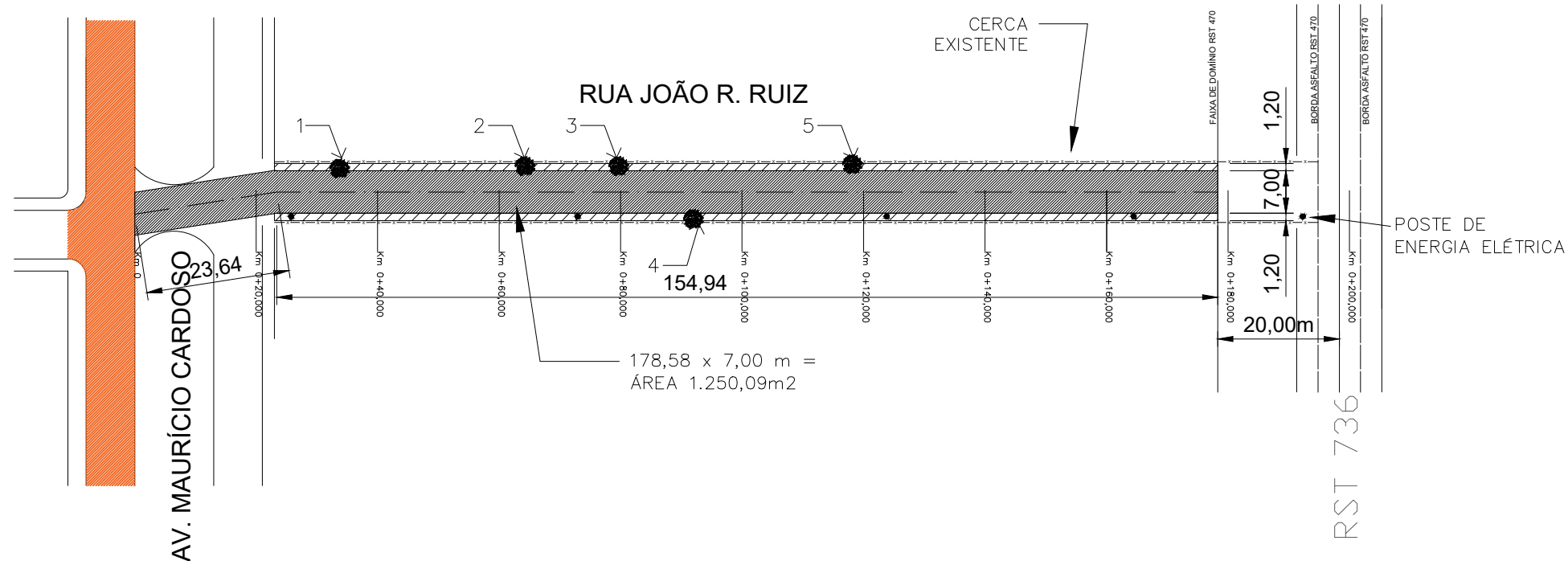
PLANTA BAIXA – PAVIMENTAÇÃO ESCALA: 1/1000
