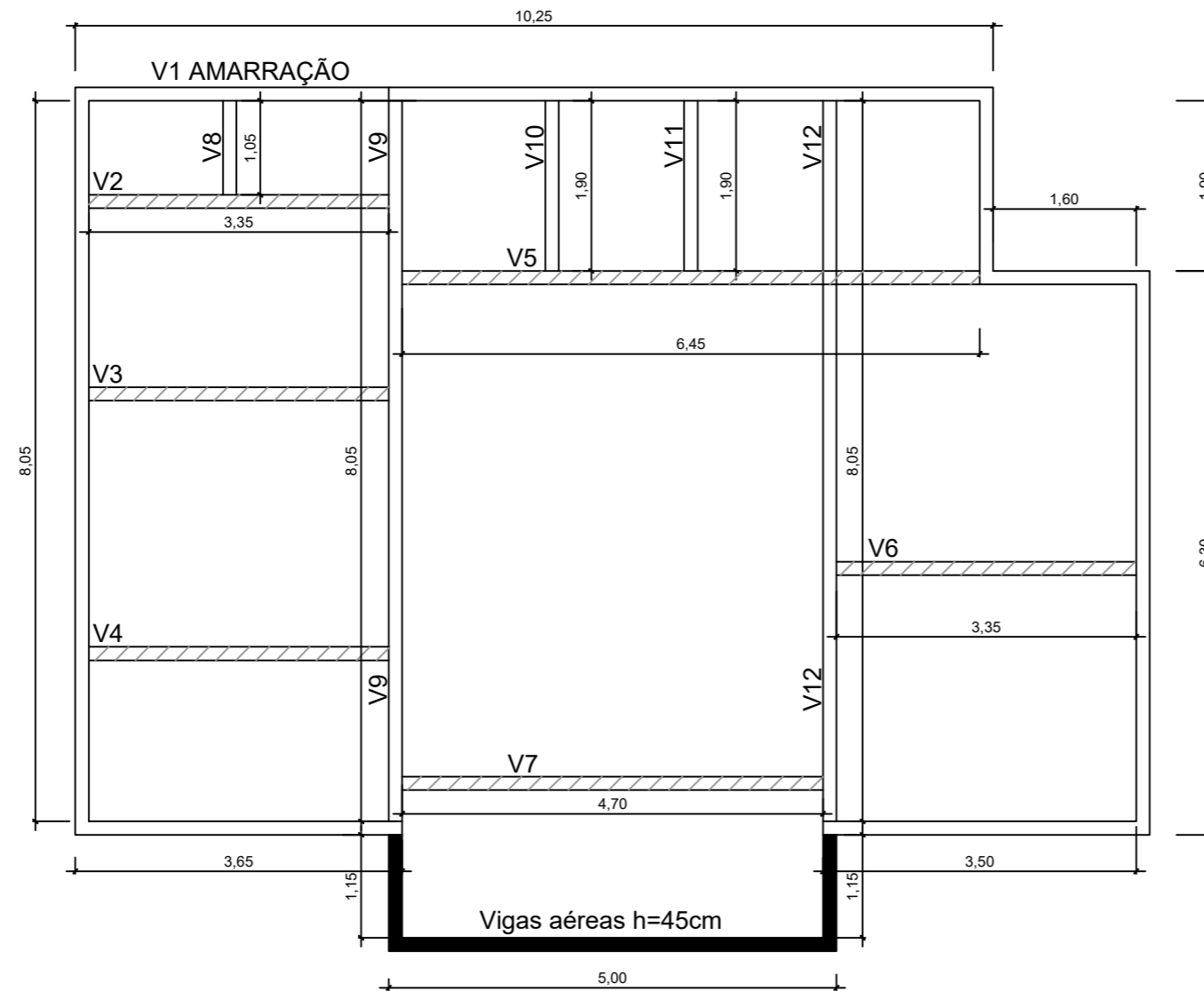
PLANTA DE VIGAS DE AMARRAÇÃO E AÉREAS ESC.:1/75
